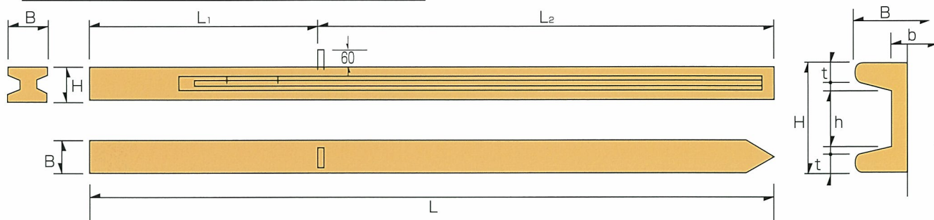
プレストレス コンクリート H 形 パイル (PCHパイル)
